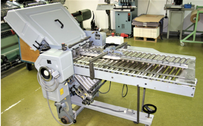
Markiereinrichtung
